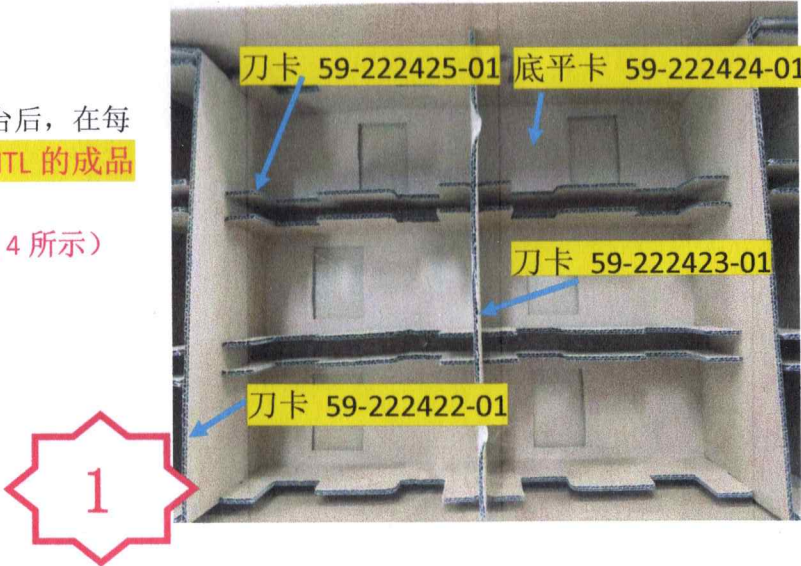
图一，如图折包材放在内箱里
