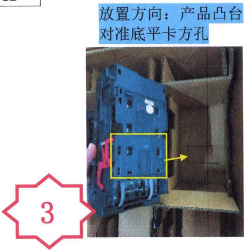
图三，出 ITL 的产品不需要装 PE 袋，如图底层放置产品需产品的凸台对准底平卡的方孔放置，底层放置 6 台产品后，在每台机上在加上 3 片隔板，共 18 片，然后在上层在放置 6 台产品
